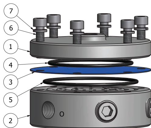
Figure A : Vue éclatée du modèle de la série GS
