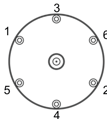
Figure B : Exemple d'ordre de serrage
