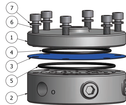
Figur A: Explosionsansicht
